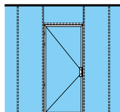
Porte battante vitrée avec imposte
