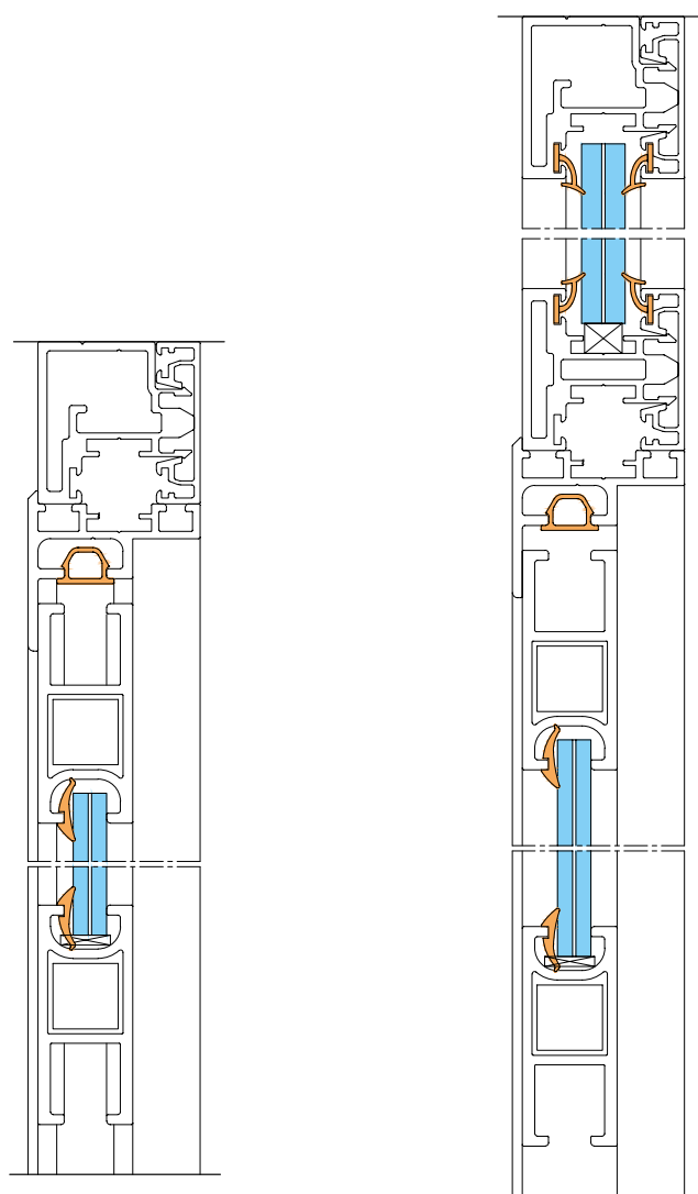
Coupe verticale
