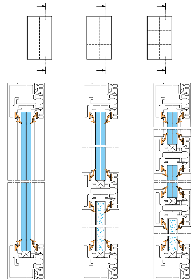
Coupe verticale
